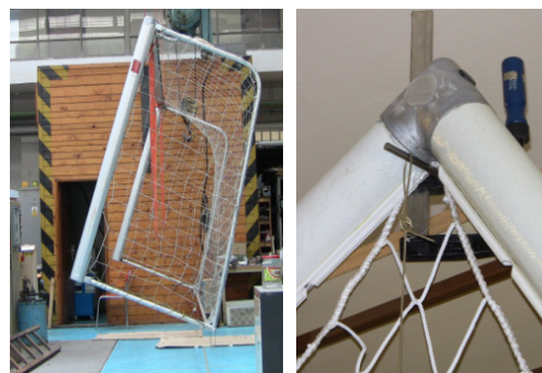
Obrázek 2 Experimentální určení polohy těžiště a momentu setrvačnosti branky
